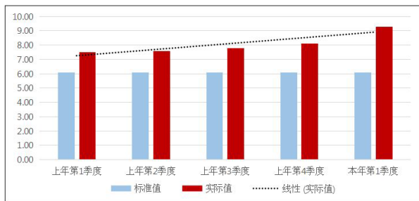
图1 近五季度主机系统油总碱值(TBN)变化 (单位:mgKOH/g)
