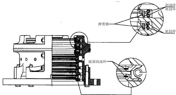
图2 扫气箱填料函结构图
